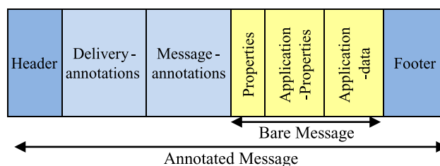
Fig. 14. AMQP message format.
